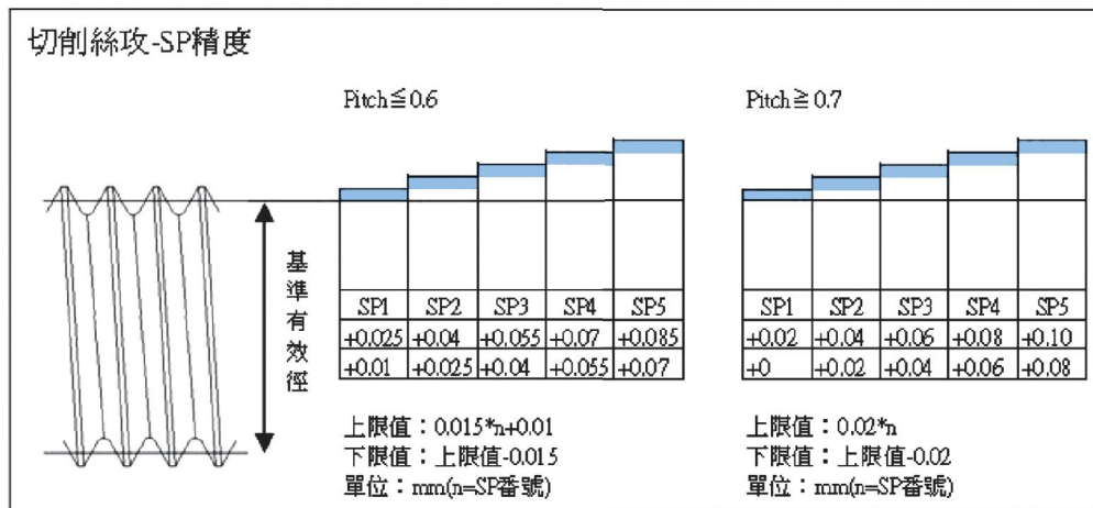
切削絲攻精度表
