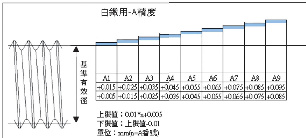
切削絲攻精度表
